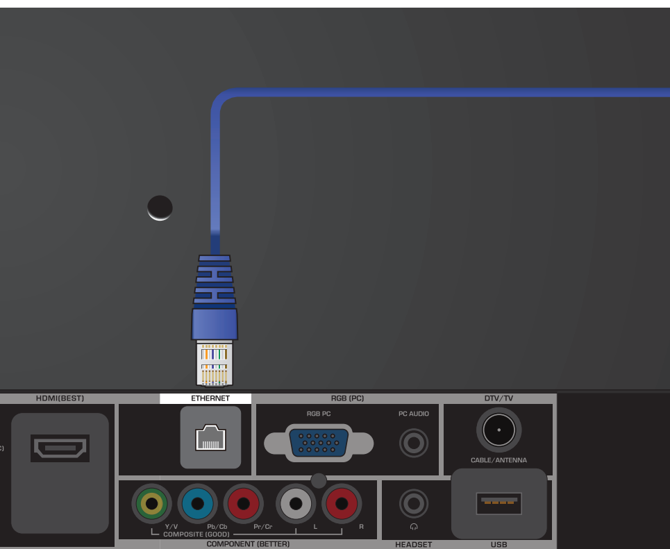
PARTE TRASERA DEL TELEVISOR
